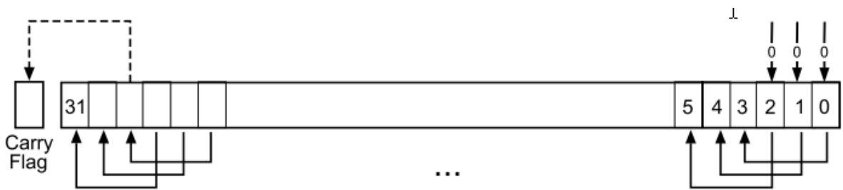
Рисунок 20 – Инструкция LSL # 3
