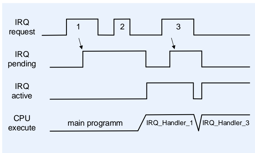
Рисунок 144 – Повторная установка запроса на прерывание в момент выполнения обработчика исключения
