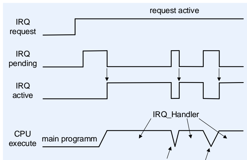
Рисунок 142 – Повторная обработка прерываний при удержании запроса от источника
