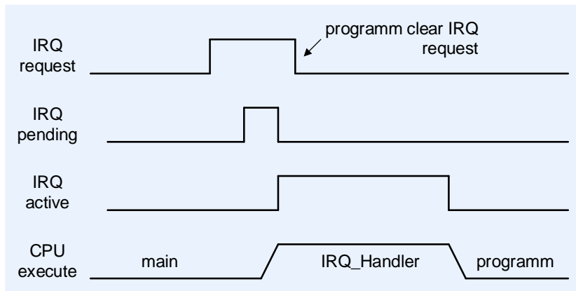
Рисунок 141 – Сброс признака отложенного прерывания, до обработки ядром
