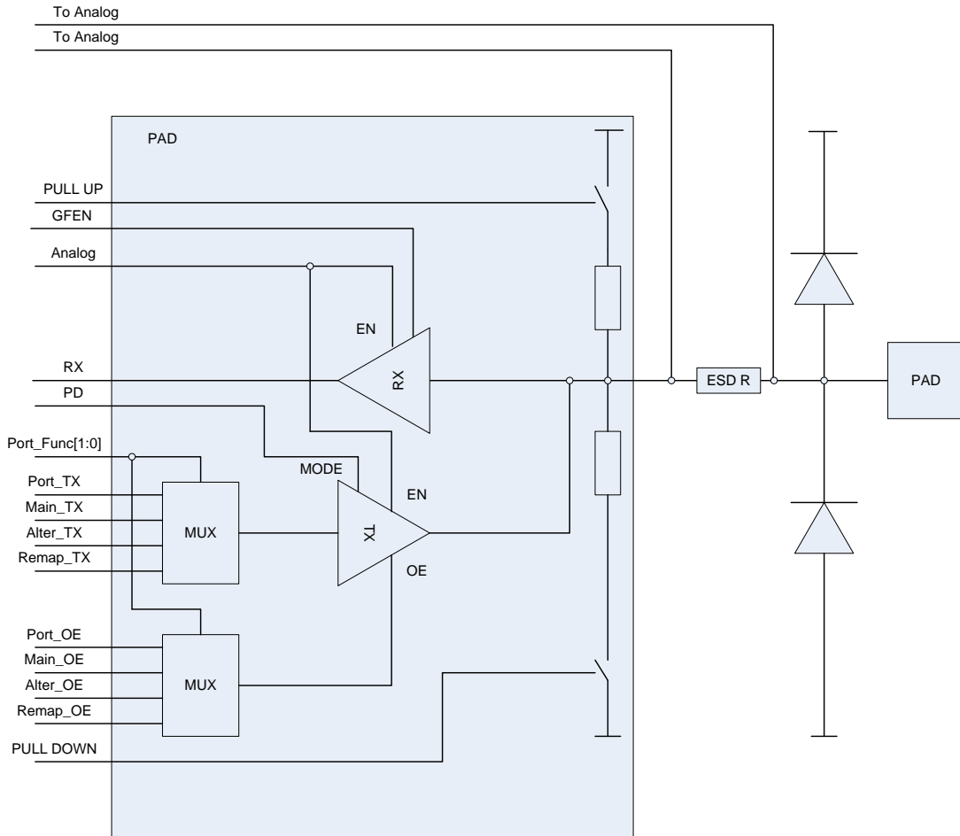
Рисунок 26 – Порты ввода/вывода
