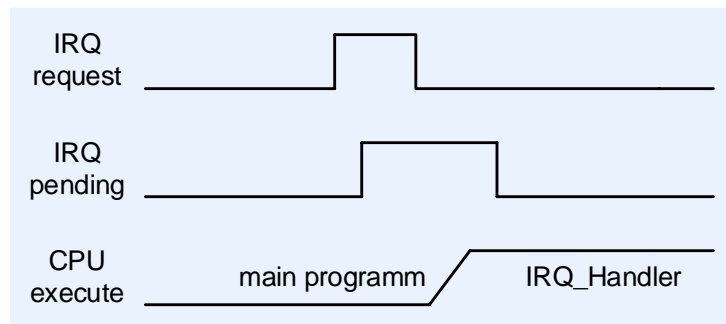
Рисунок 139 – Выставление отложенного запроса на прерывание и последующая его обработка
