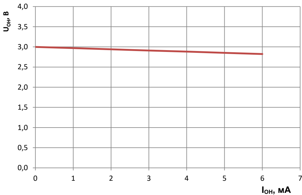
Рисунок 148 – Зависимость выходного напряжения высокого уровня от выходного тока высокого уровня при напряжении питания 3,0 В
