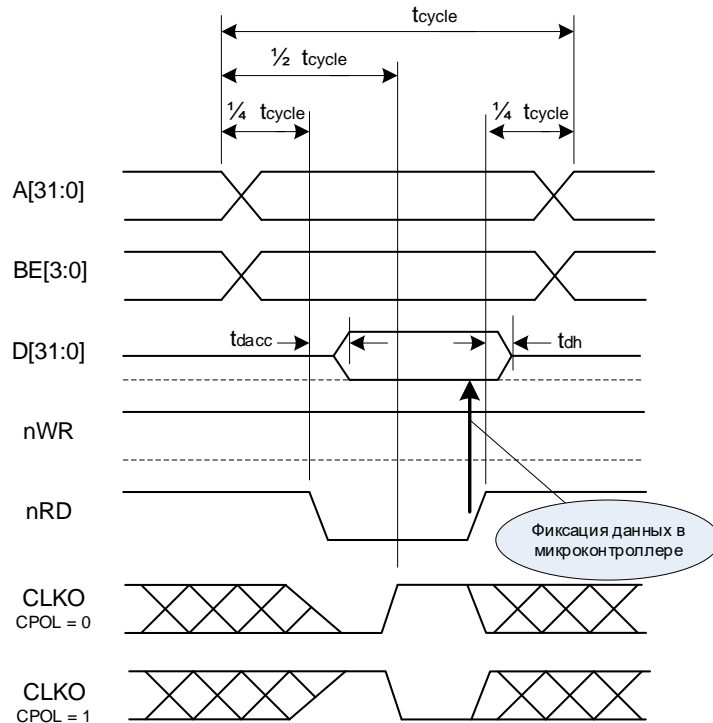
Рисунок 29 – Диаграмма чтения
