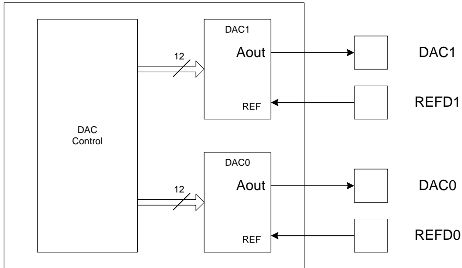
Рисунок 94 – Структурная схема контроллера ЦАП
