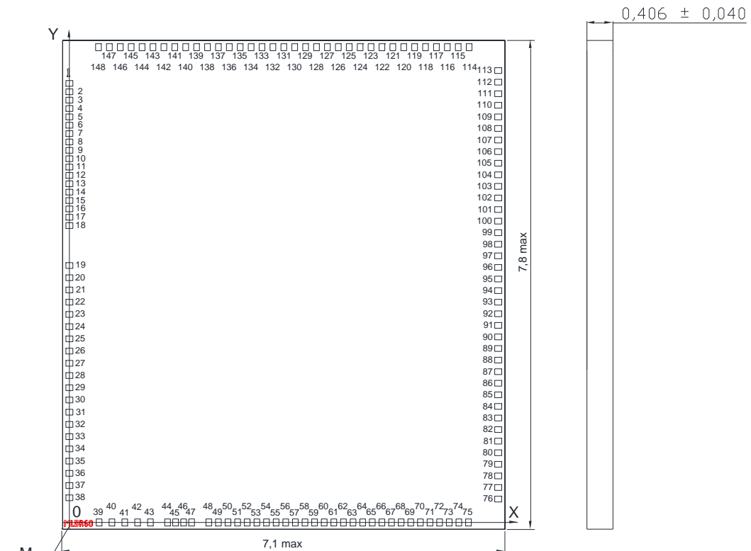
Рисунок 151 – Габаритный чертеж микросхемы в корпусе с формованными выводами
