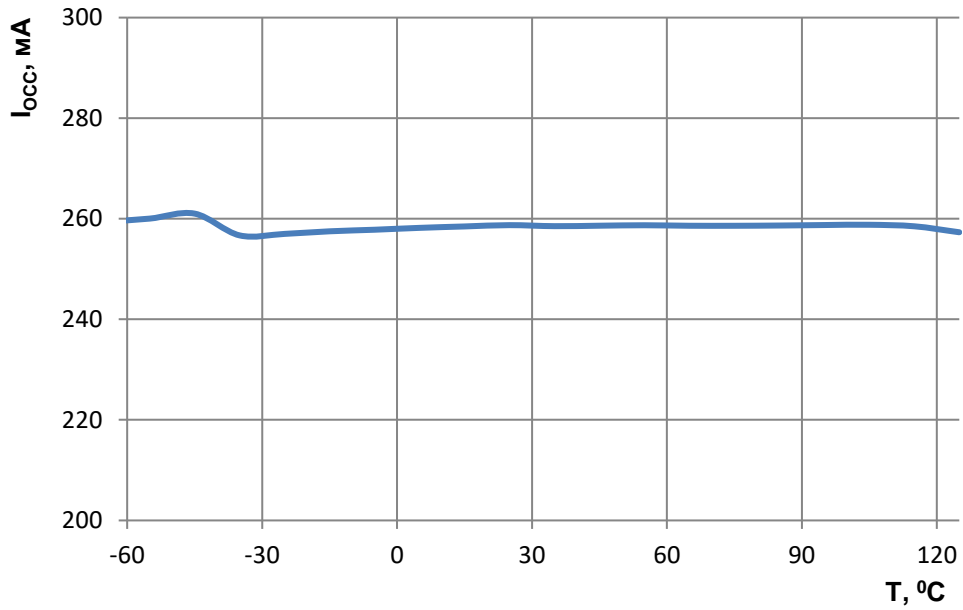
Рисунок 145 – Зависимость динамического тока потребления от температуры при: f_c = 144 МГц
