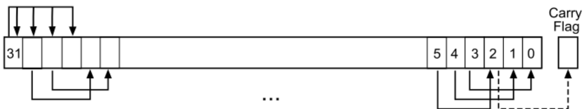
Рисунок 18 – Инструкция ASR # 3
