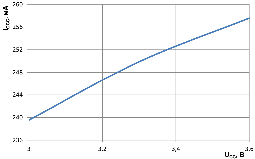
Рисунок 146 – Зависимость динамического тока потребления от напряжения питания
