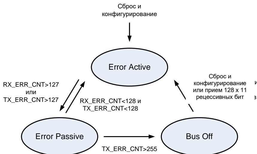
Рисунок 54 – Счетчики ошибок
