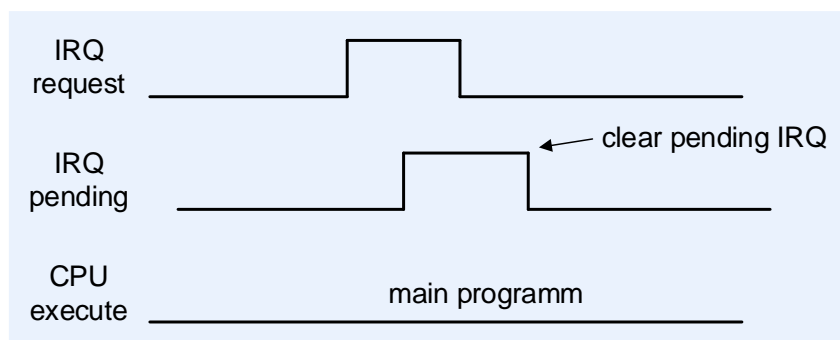
Рисунок 140 – Сброс признака отложенного прерывания, до обработки ядром
