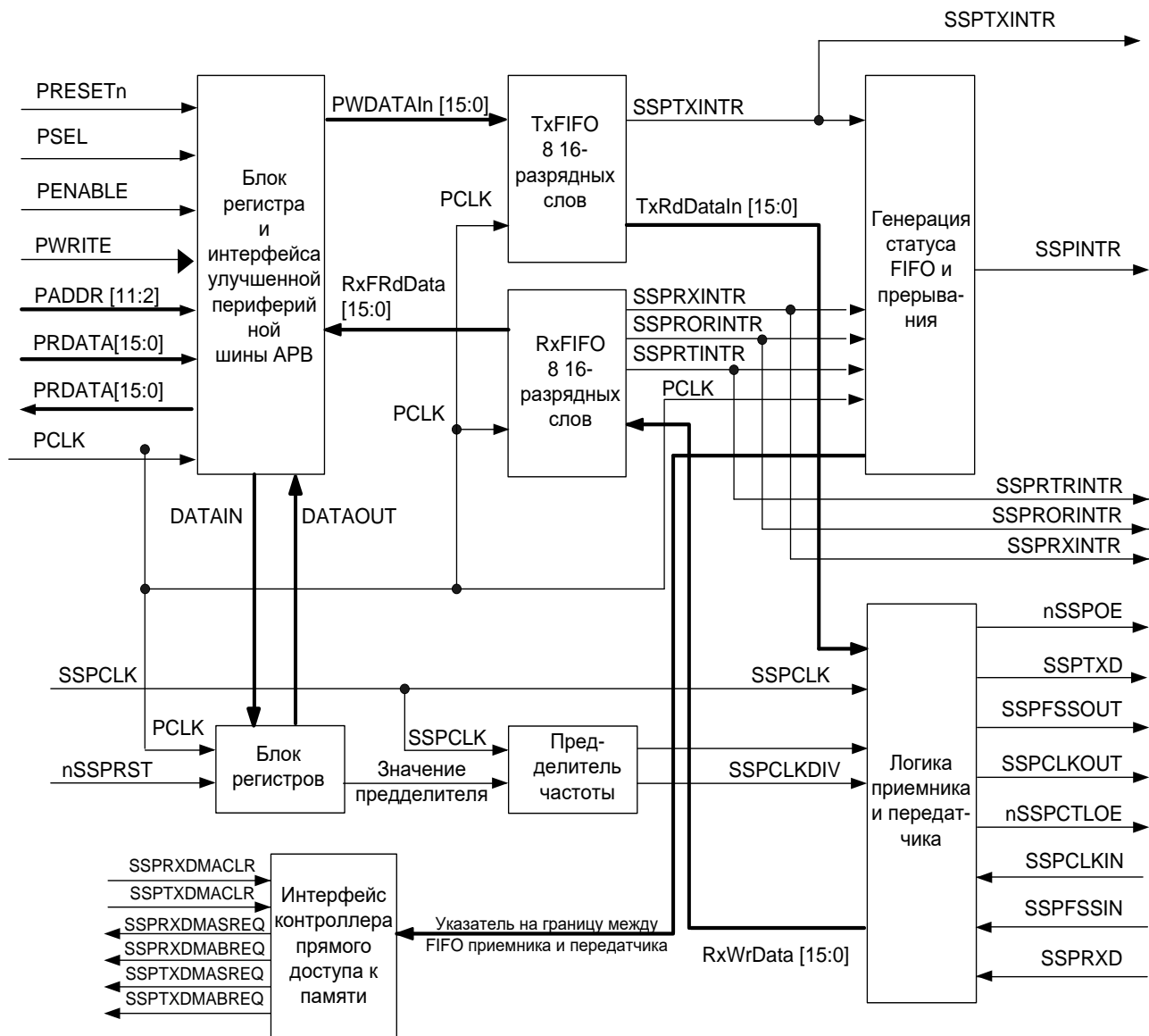
Рисунок 99 – Структурная схема модуля SSP
