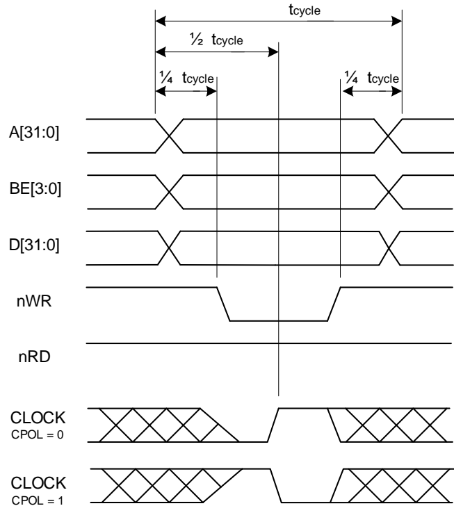
Рисунок 28 – Диаграмма записи
