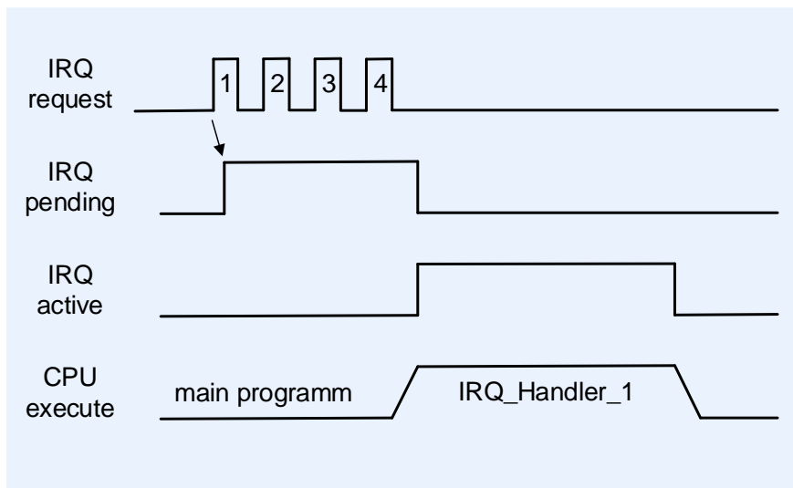
Рисунок 143 – Многократная установка снятие запроса IRQ request
