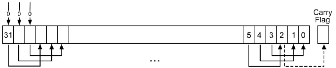
Рисунок 19 – Инструкция LSR # 3
