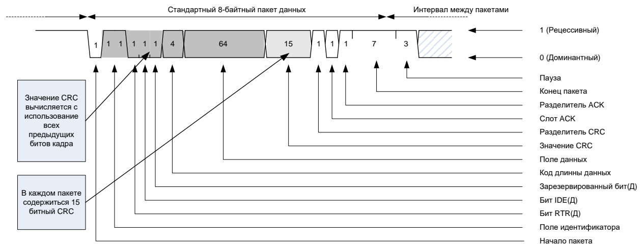
Рисунок 51 – Контроль CRC
