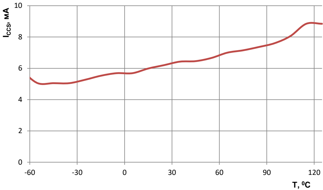
Рисунок 147 – Зависимость статического тока потребления в режиме покоя (регулятор напряжения выключен) от температуры при разном напряжении
