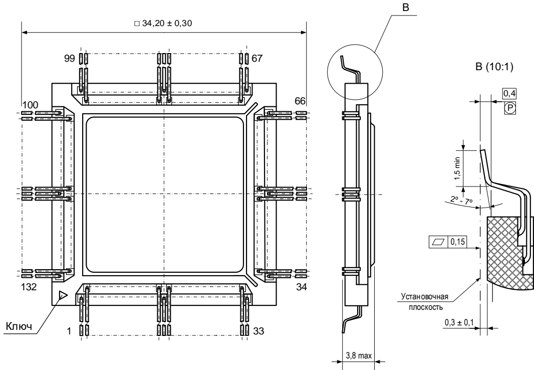
Рисунок 151 – Габаритный чертеж микросхемы в корпусе с формованными выводами
