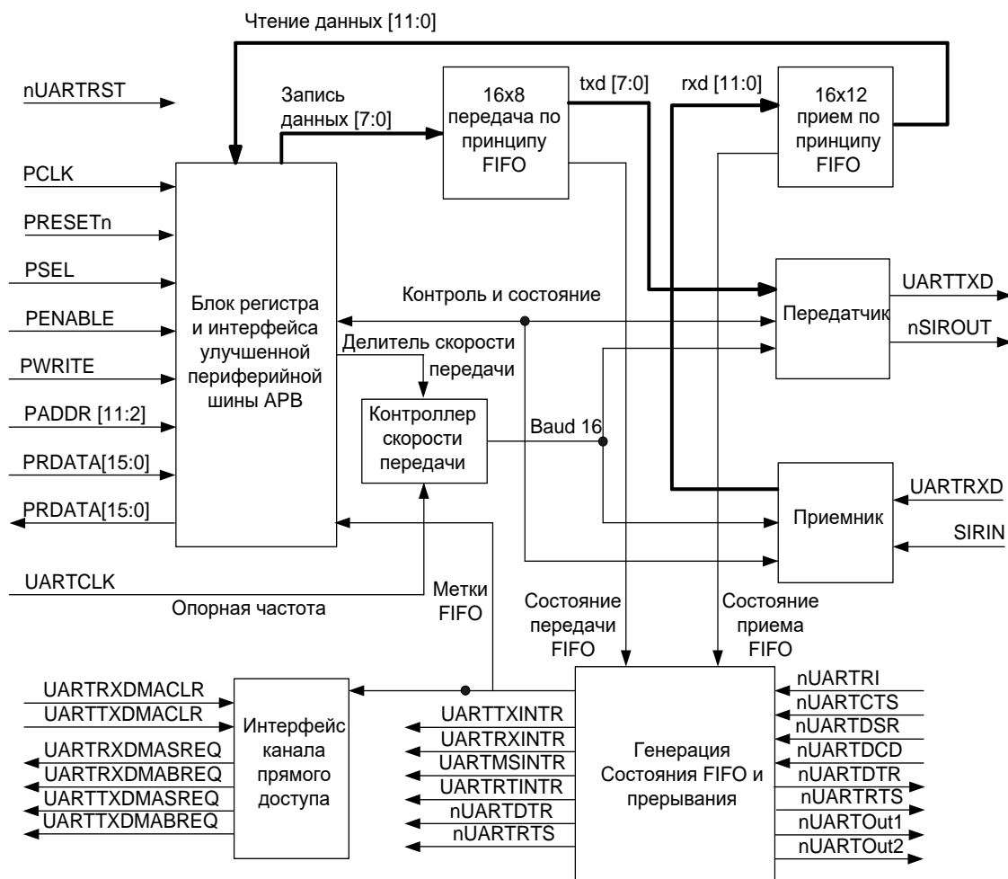
Рисунок 115 – Блок-схема универсального асинхронного приёмопередатчика (UART)
