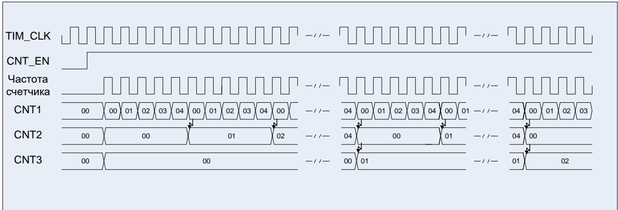
Рисунок 73 – Диаграммы работы трех таймеров в каскаде DIR_1, DIR_2, DIR_3 = 0; EVENT_SEL_1 = 0000, EVENT_SEL_2 = 0001, EVENT_SEL_3 = 0010; CNT_MODE_1, CNT_MODE_2, CNT_MODE_3 = 00;
