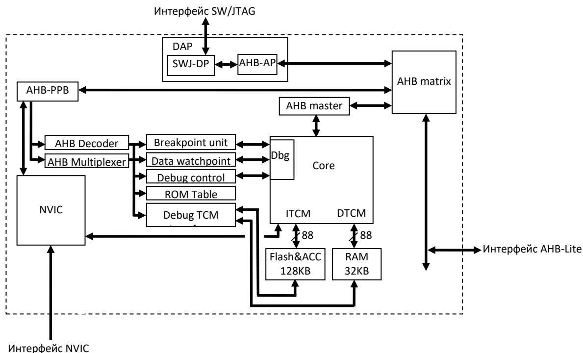
Рисунок 16 – Структурная блок-схема процессорного ядра
