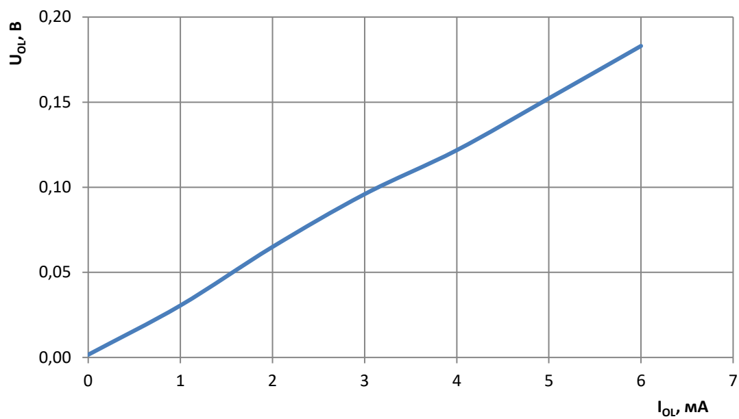
Рисунок 149 – Зависимость выходного напряжения низкого уровня от выходного тока низкого уровня при напряжении питания 3,0 В
