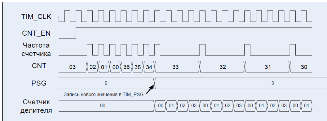
Рисунок 70 – Диаграммы работы счетчика: счет вниз (CNT_MODE = 00, EVENT_SEL = 0000, DIR = 1)
